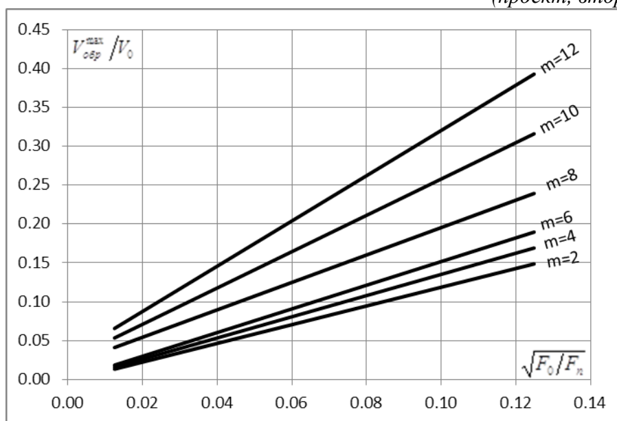
Рисунок Ж.2 – Зависимость максимальной скорости в обратном потоке от параметра
