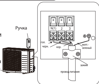
соединение внутреннего и наружного блоков
