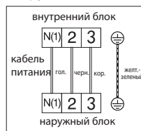
соединение внутреннего и наружного блоков
