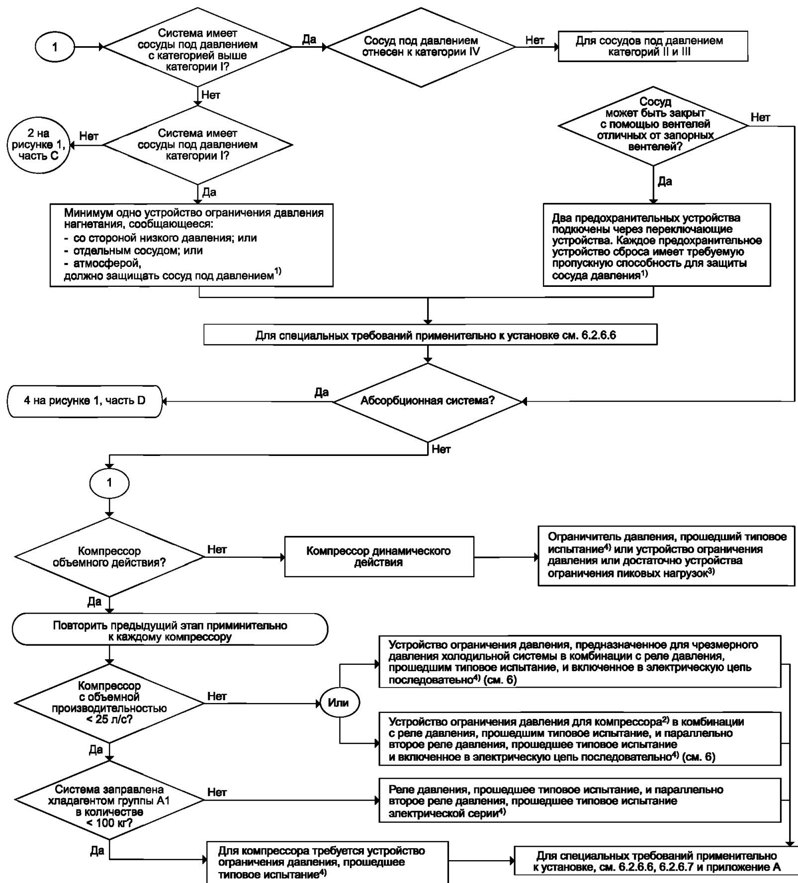
Рисунок 1, часть В — Защита холодильной системы от чрезмерного давления
