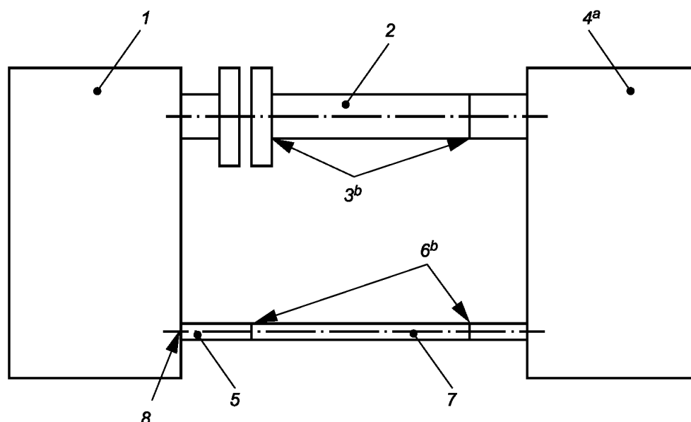
Рисунок В.1 — Соединения оборудования под давлением
