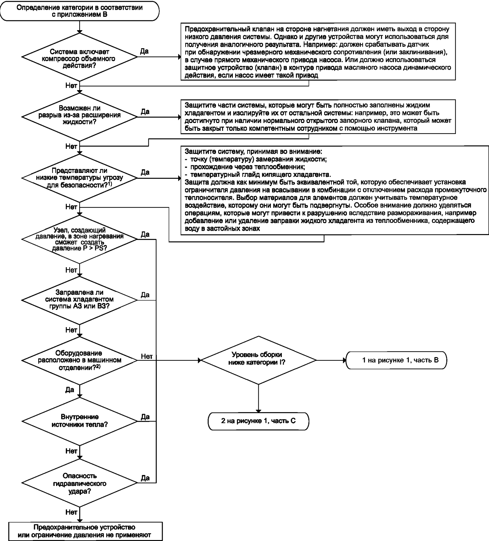
Рисунок 1, часть А — Защита холодильной системы от чрезмерного давления
