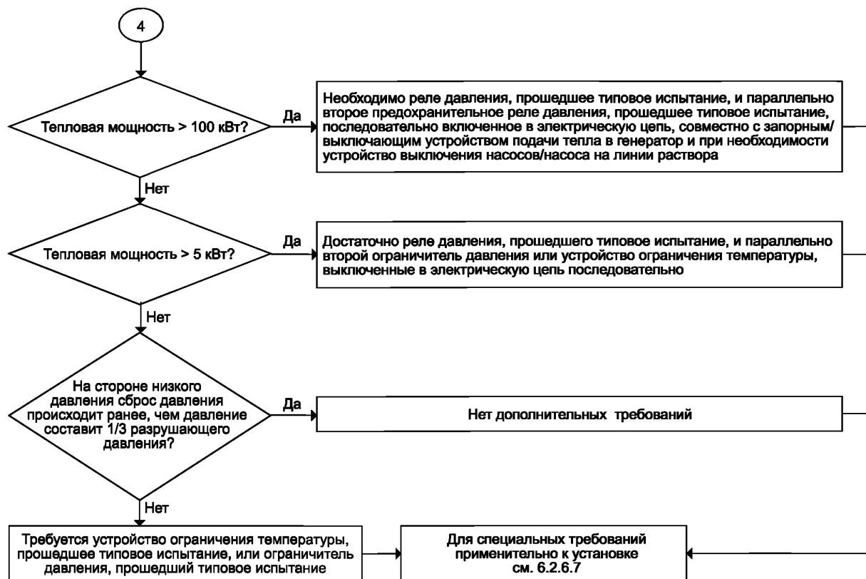
Рисунок 1, часть D — Защита системы охлаждения от чрезмерного давления
