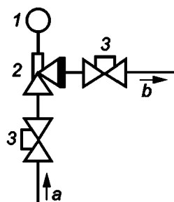
Рисунок F.1 — Установка предохранительных клапанов, оснащенных устройством мониторинга их герметичности
