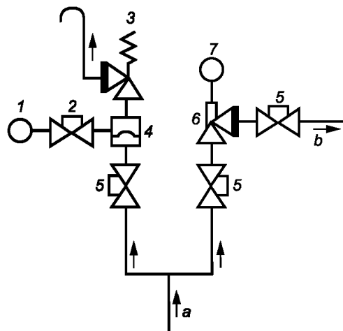
Рисунок F.3 — Перепускной клапан, не зависящий от противодействия, для защиты сосудов на стороне низкого давления от расширения жидкости и/или внешнего теплового воздействия
