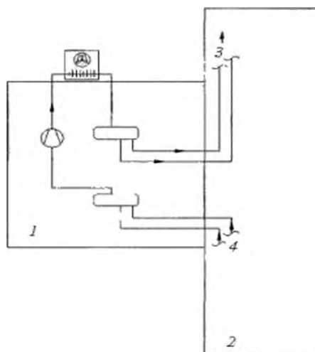
1 – машинное отделение (специальное машинное отделение); 2 – помещение, содержащее холодопотребляющий объект; 3 – жидкостные трубопроводы с хладагентом (к испарителям); 4 – трубопроводы всасывания (из испарителей)
