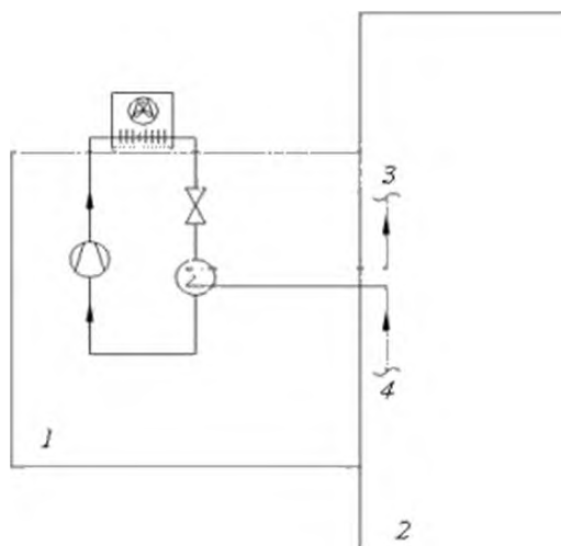
1 – машинное отделение (специальное машинное отделение); 2 – помещение, содержащее холодопотребляющий объект; 3 – трубопроводы подачи теплоносителя; 4 – трубопроводы возврата теплоносителя
