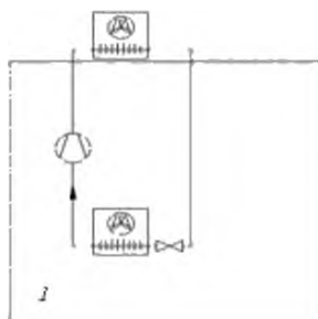
1 — помещение, содержащее холодопотребляющий объект
