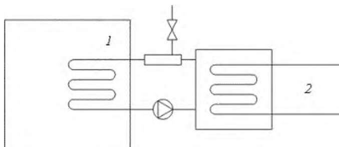
Рисунок 2с – Закрытая промежуточная система с вытяжкой
