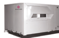
Спиральные компрессоры Sanyo, Danfoss R410a DR-40-110GUS(T)AF 41-108 кВт
